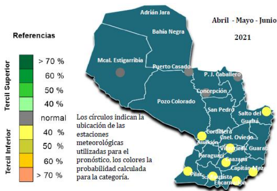
Figura 7: . Pronóstico de Precipitación trimestre . AMJ 2021.
