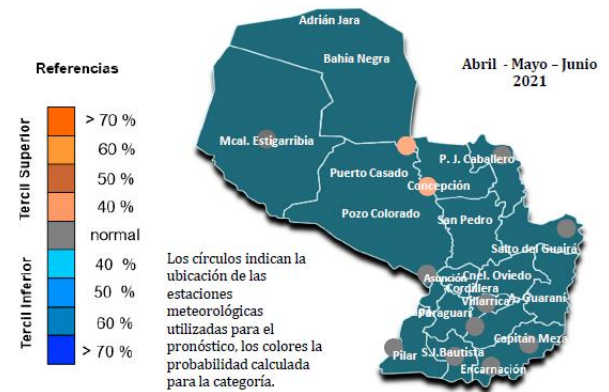
Figura 9: Pronóstico de temperatura mínima media. AMJ 2021
