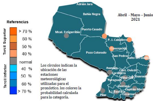
Figura 8: Pronóstico de temperatura máxima media. AMJ 2021
